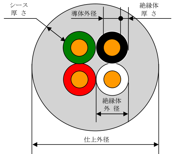
【構造断面図】
