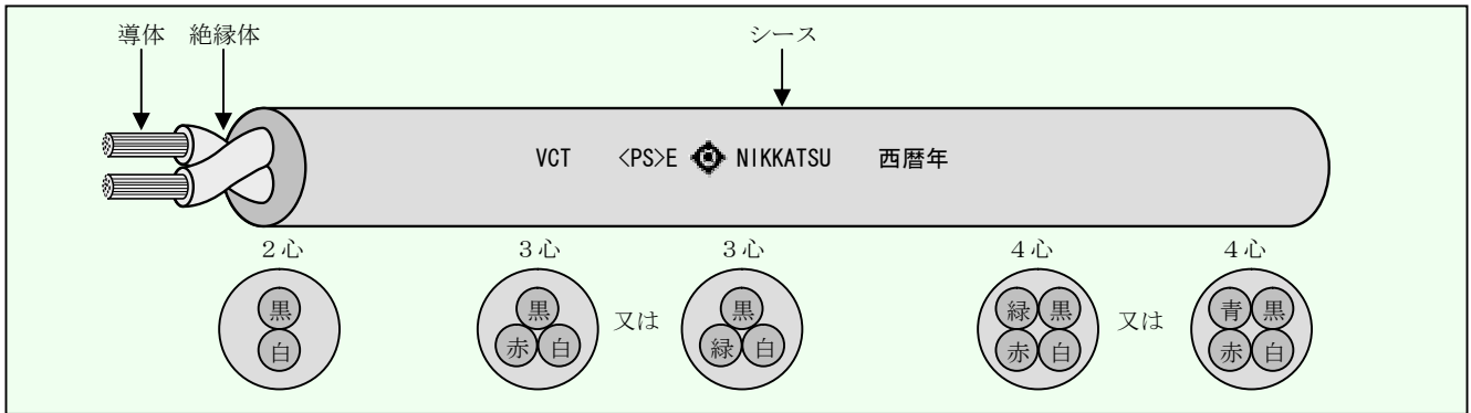
【構造図】
