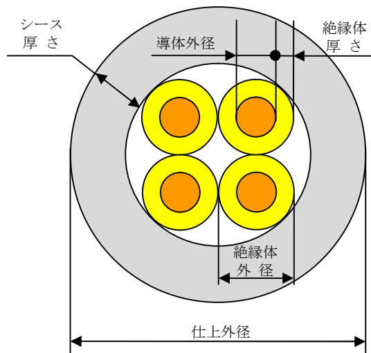
【構造断面図】
